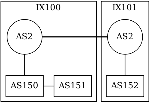
图 1: 任务 3 的互联网仿真器
