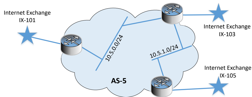
图 3: AS-5 的网络图
