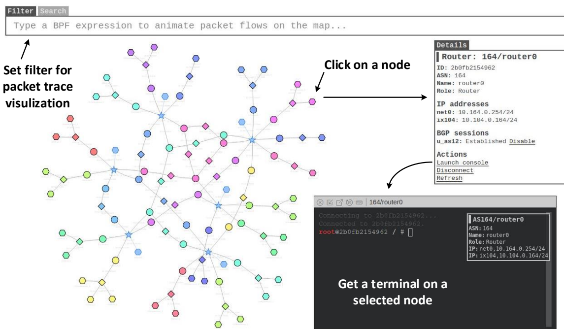
图 1: SEED 互联网仿真器
