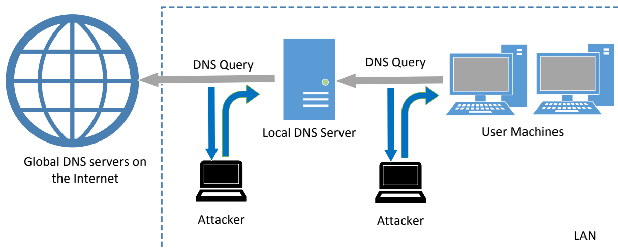
图 2: 本地 DNS 投毒攻击
