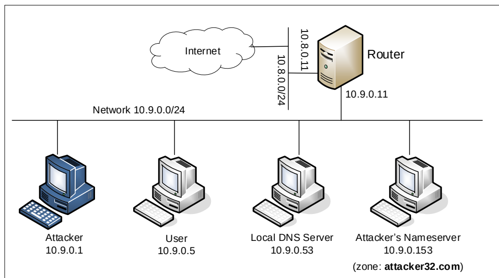
图 1: 实验环境设置
