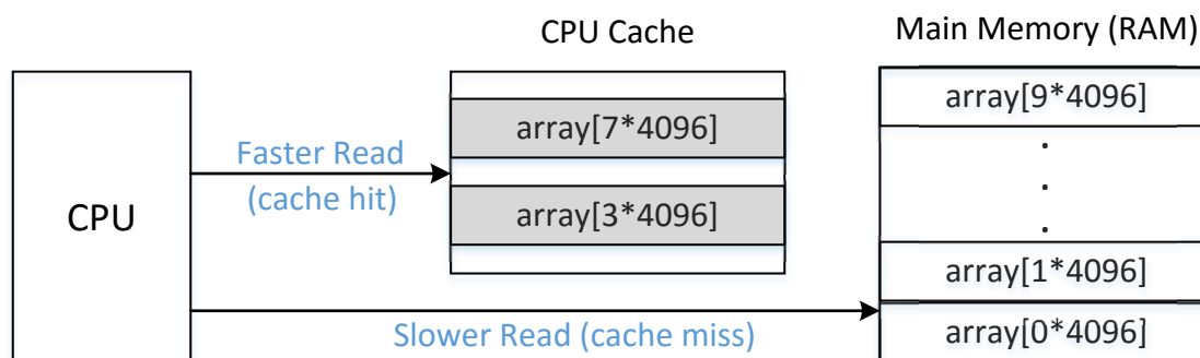
图 1: 缓存命中与未命中
