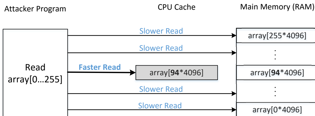
图 2：侧信道攻击的示意图
