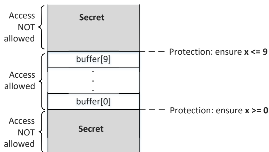
图 4: 实验配置：缓冲区和受保护的秘密
