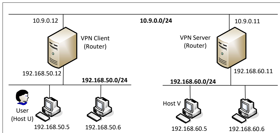
图 2: 两个专用网络之间的 VPN
