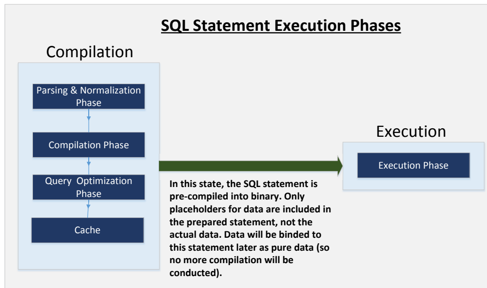
图 3: Prepared 语句的工作流程
